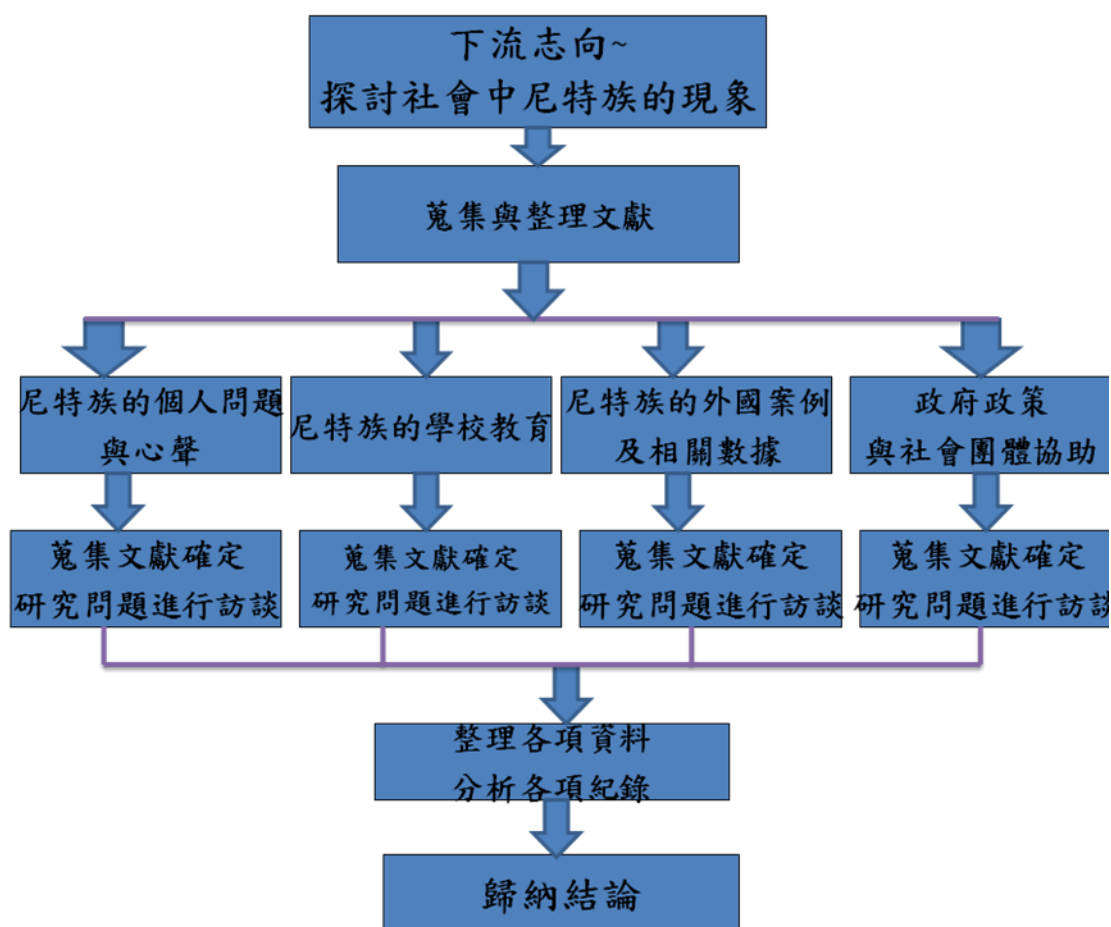
圖 3-1：研究架構
